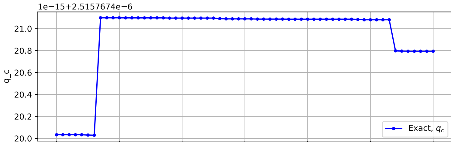
Trajectory No. 2369
