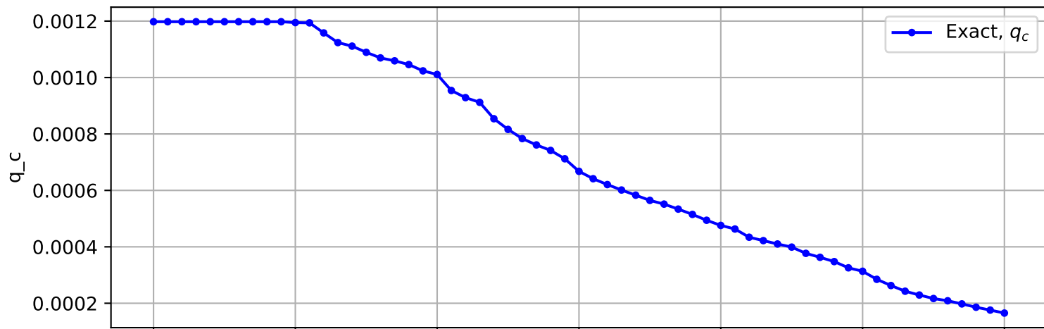
Trajectory No. 2374
