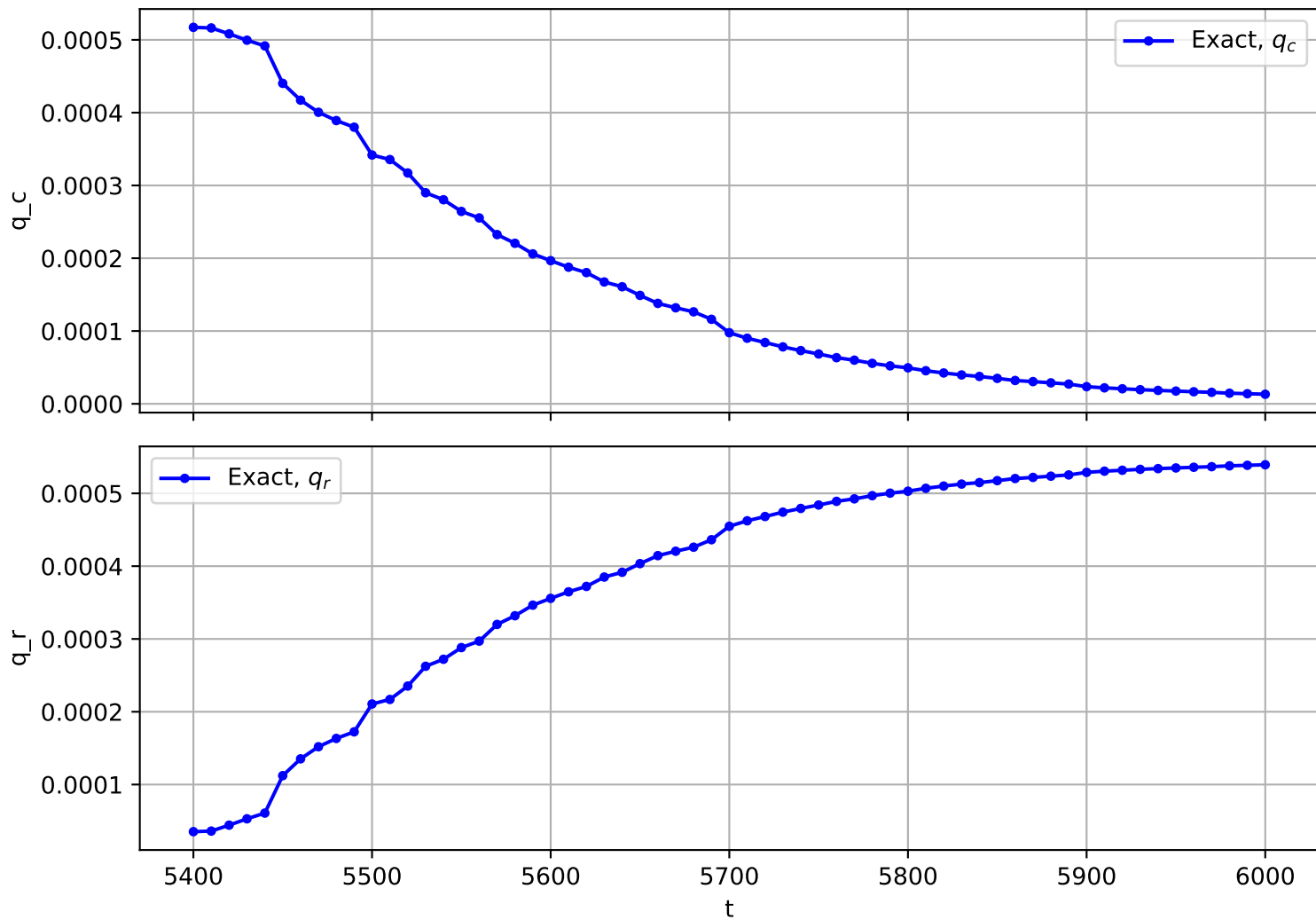
Trajectory No. 2406
