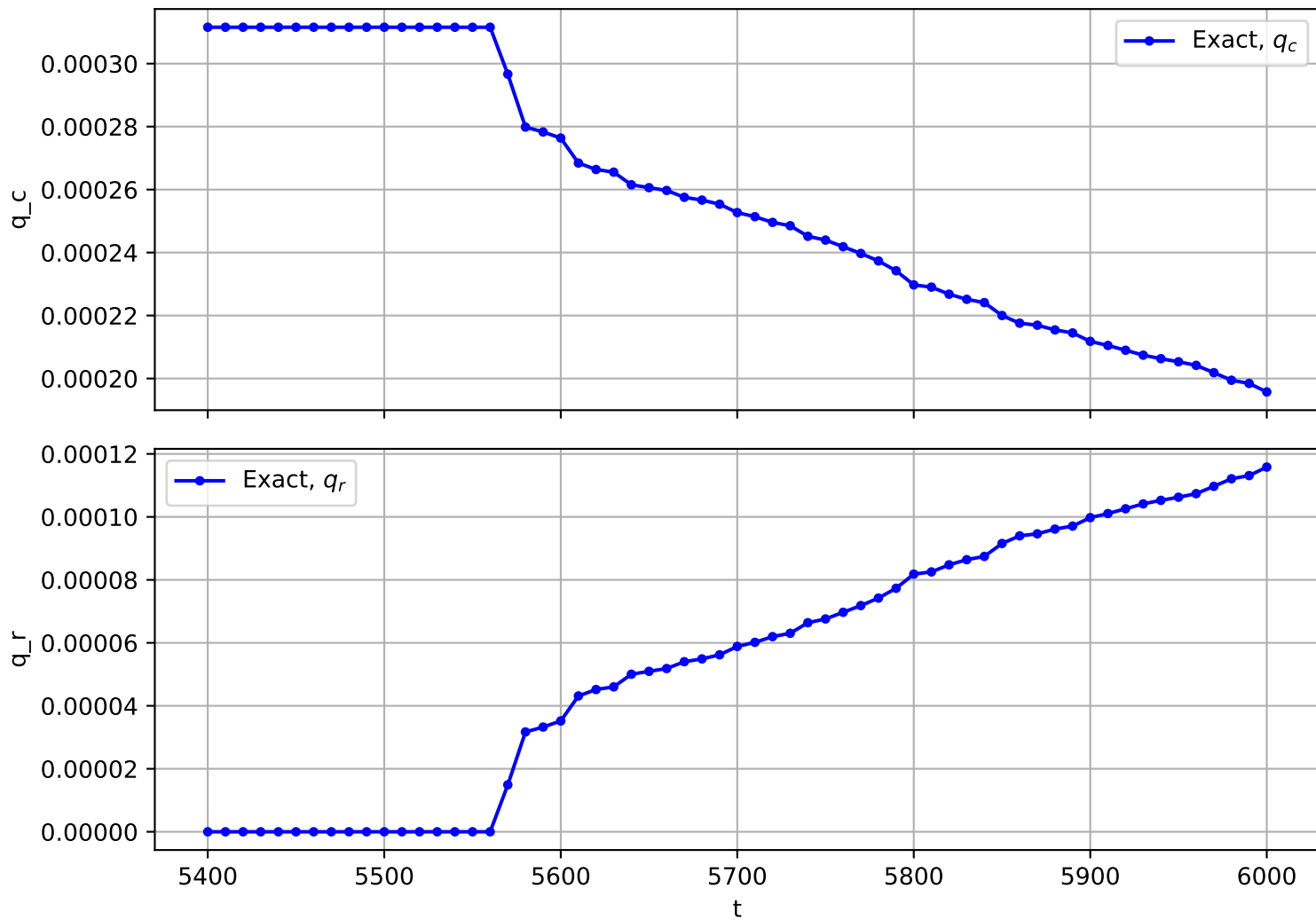
Trajectory No. 2429
