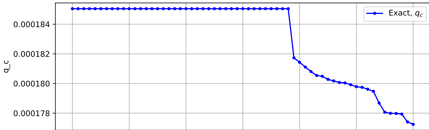
Trajectory No. 2436
