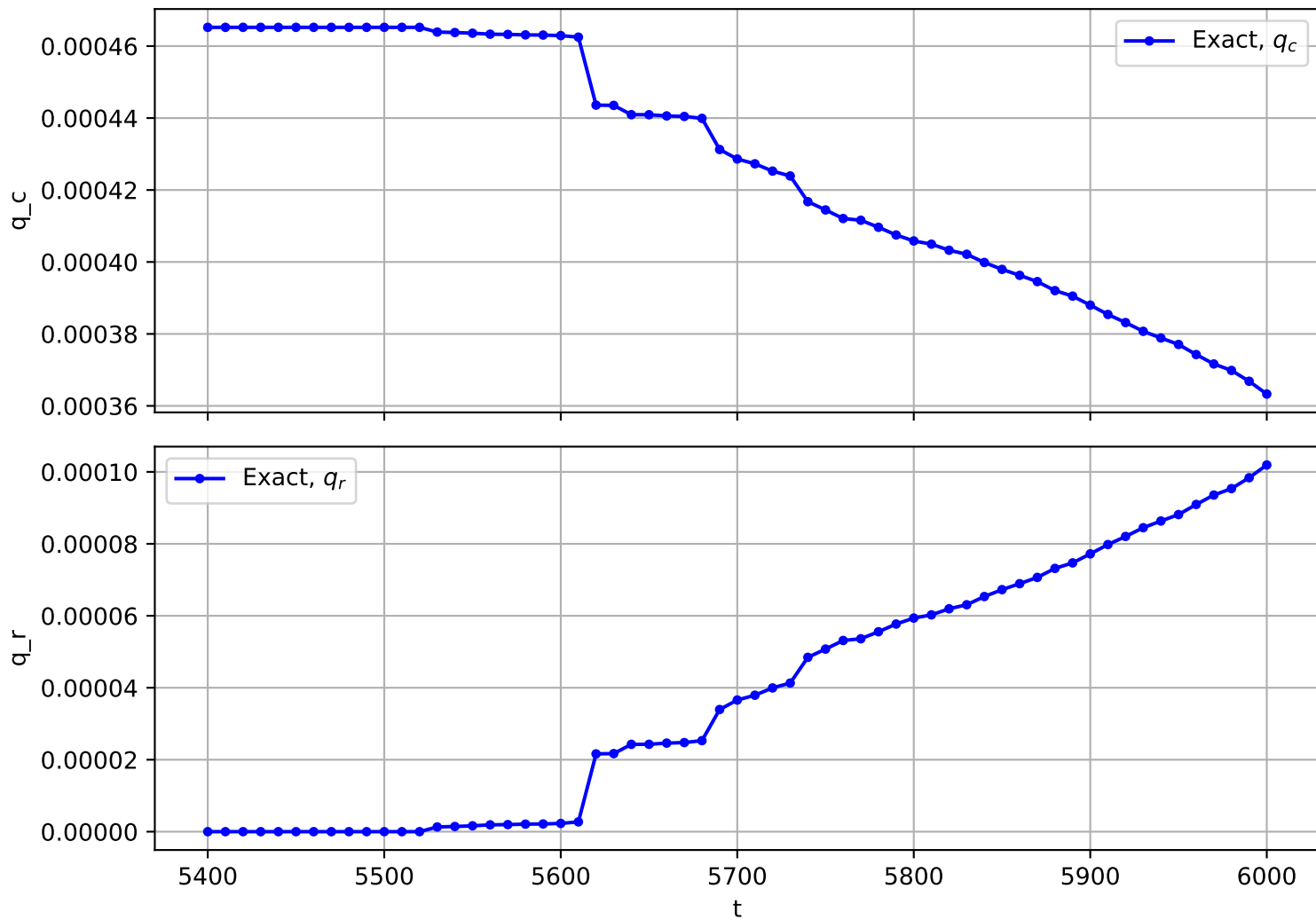
Trajectory No. 2439
