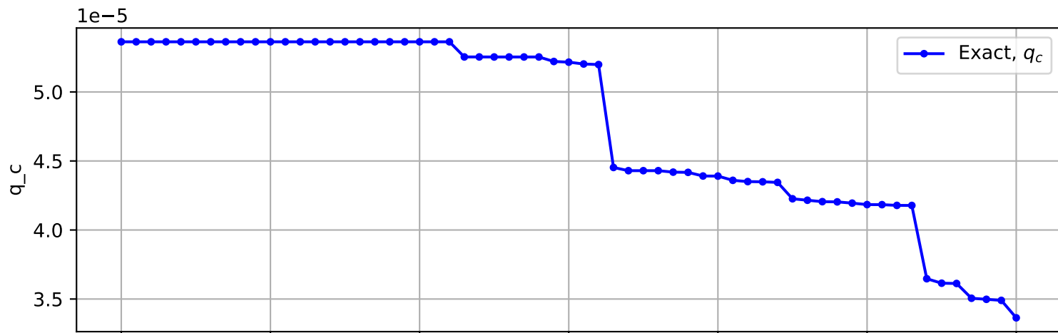
Trajectory No. 2446
