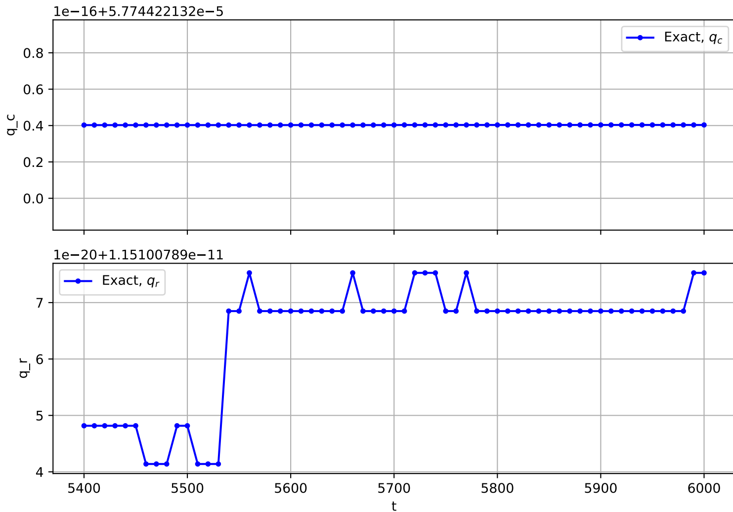
Trajectory No. 2453
