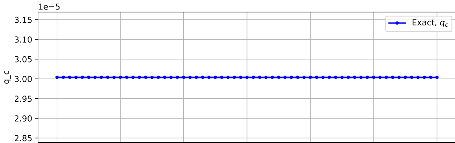
Trajectory No. 2457
