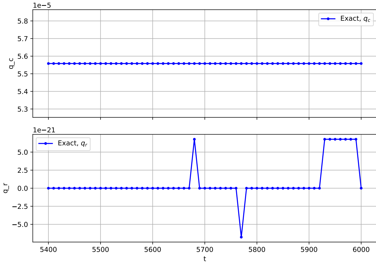
Trajectory No. 2461
