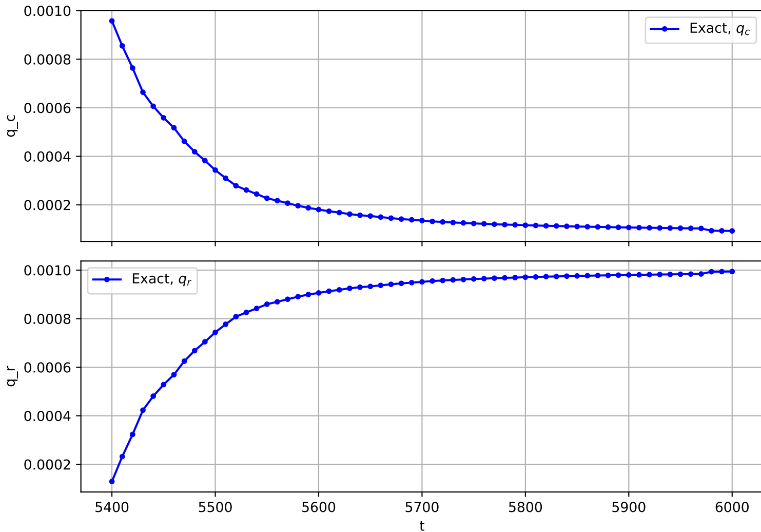
Trajectory No. 2517
