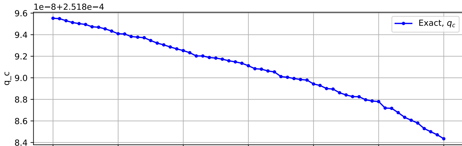
Trajectory No. 2533
