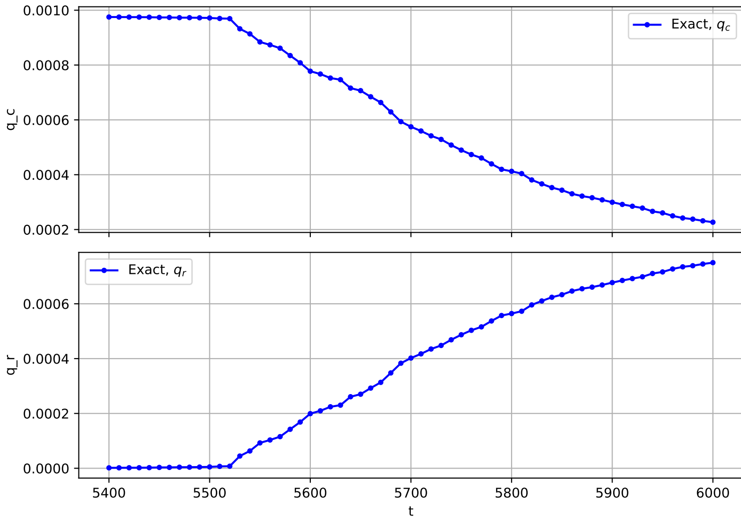
Trajectory No. 2537
