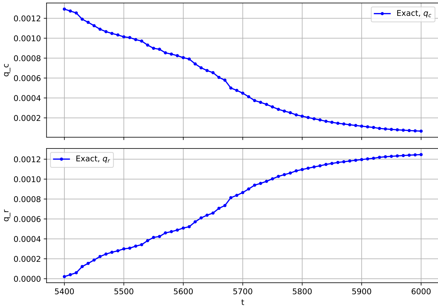
Trajectory No. 2619
