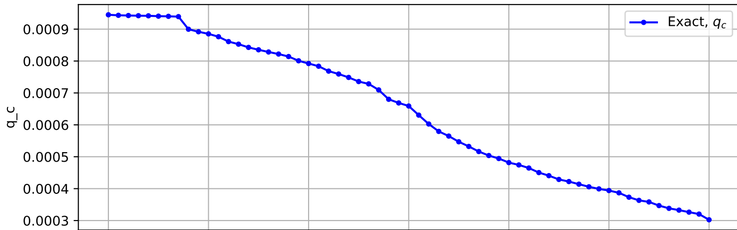
Trajectory No. 2643
