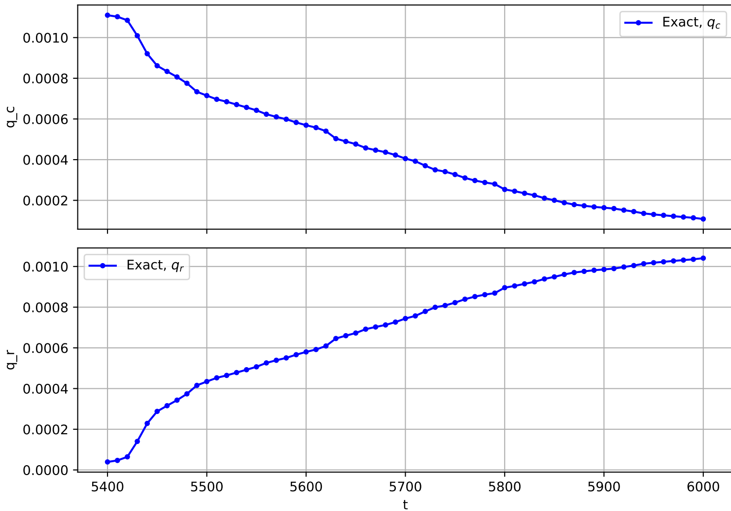
Trajectory No. 2651
