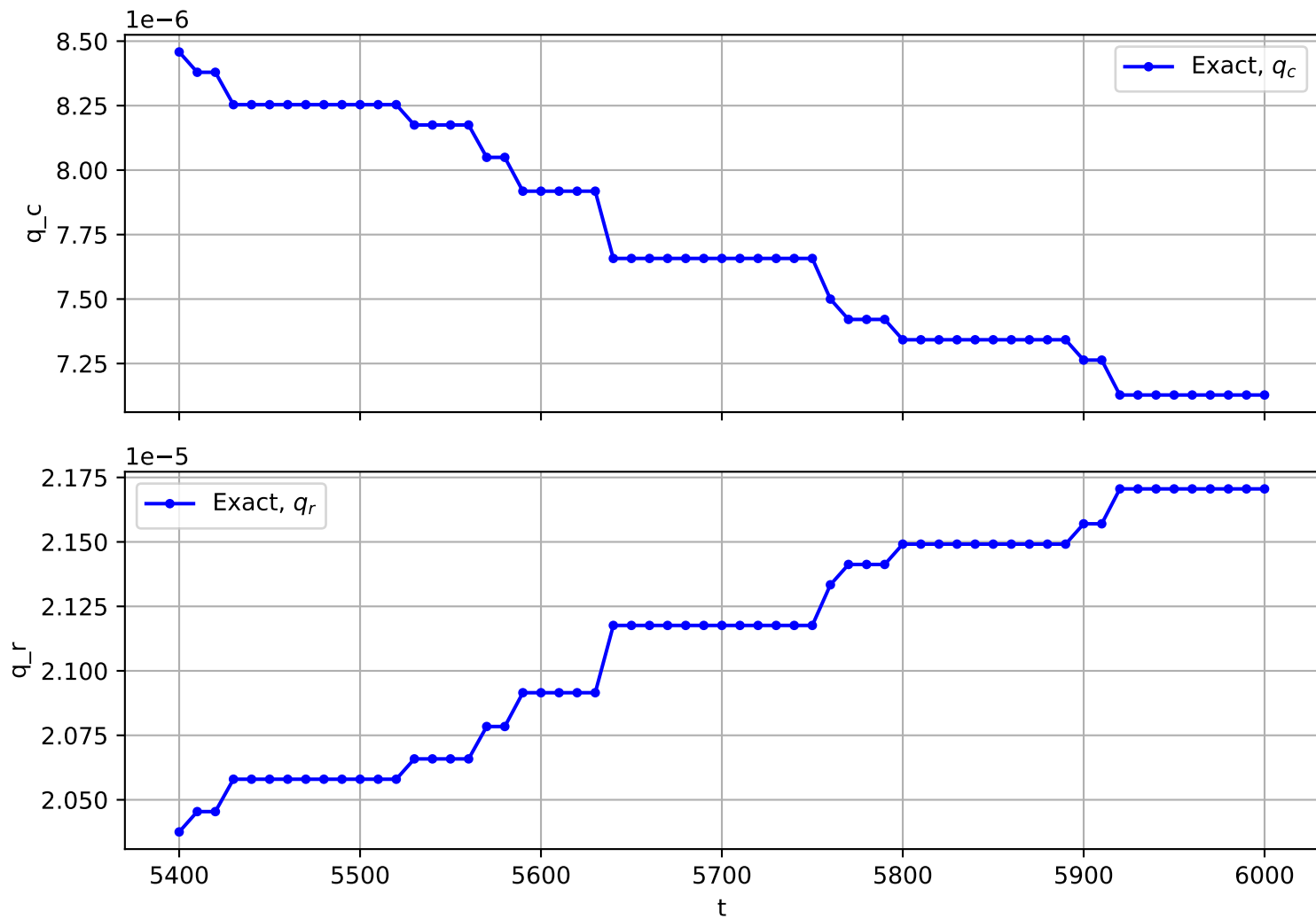
Trajectory No. 2726
