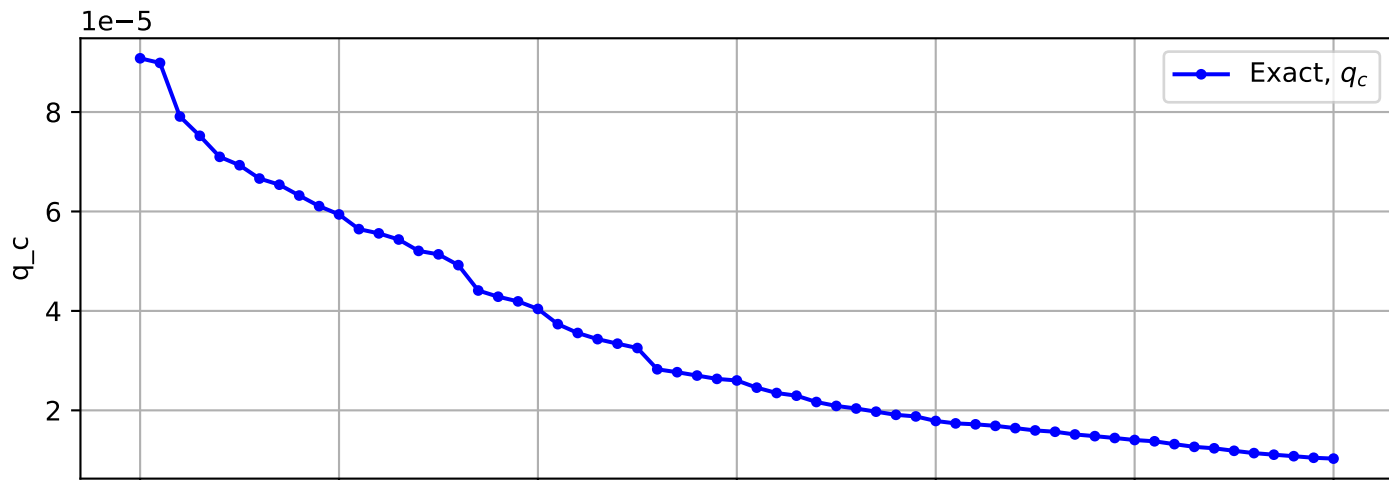
Trajectory No. 2731
