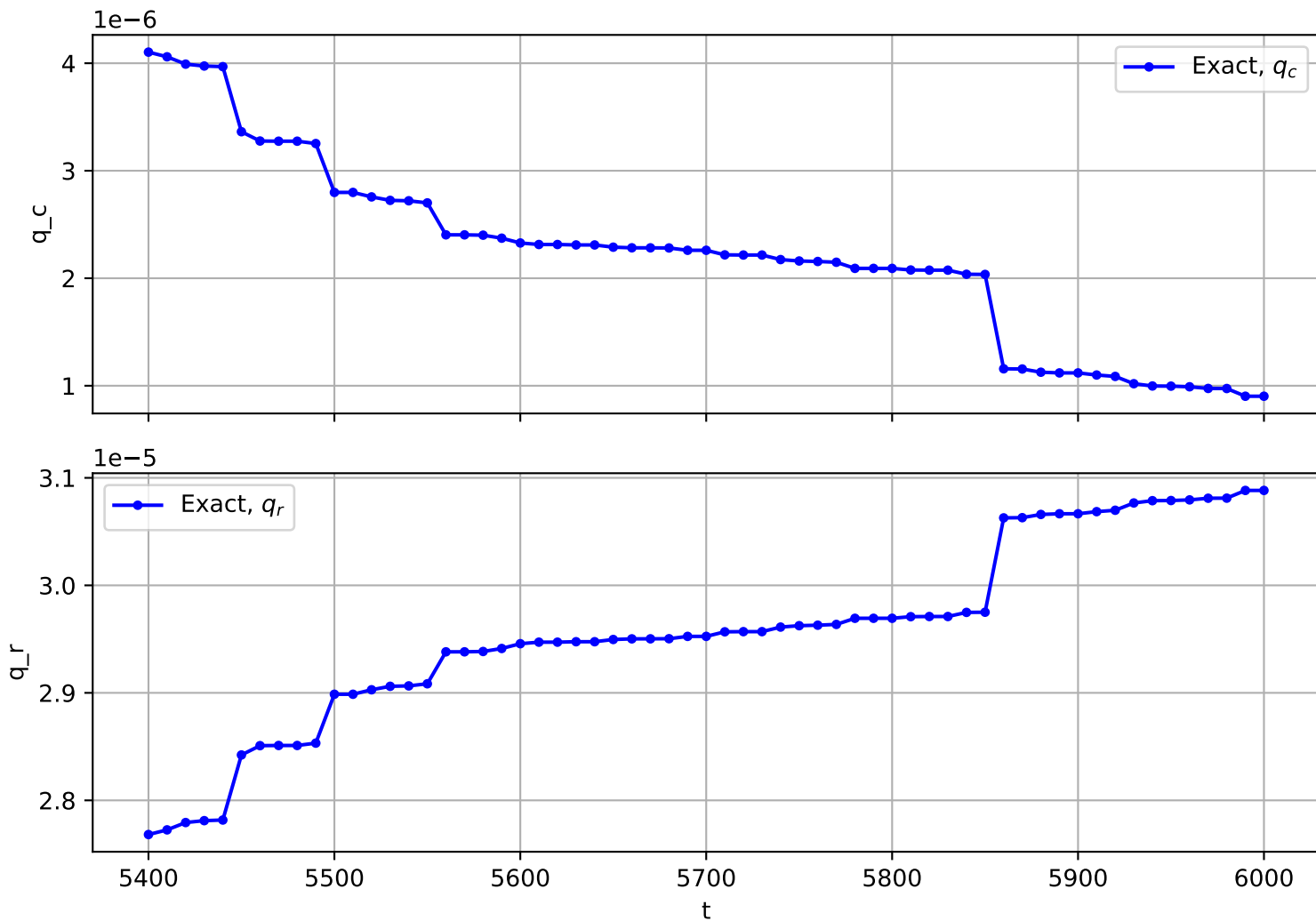
Trajectory No. 2750
