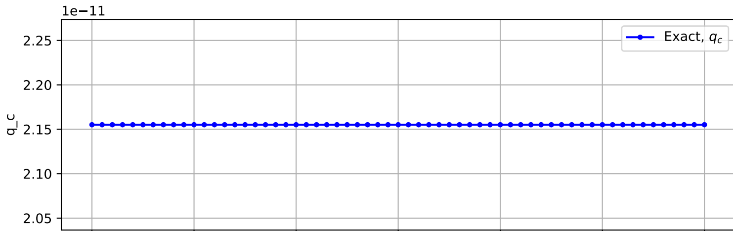
Trajectory No. 2834
