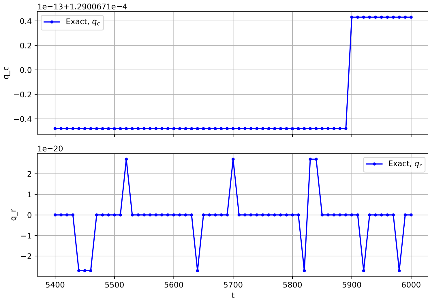
Trajectory No. 2918
