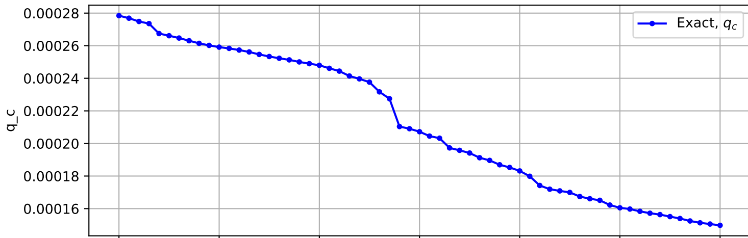
Trajectory No. 292
