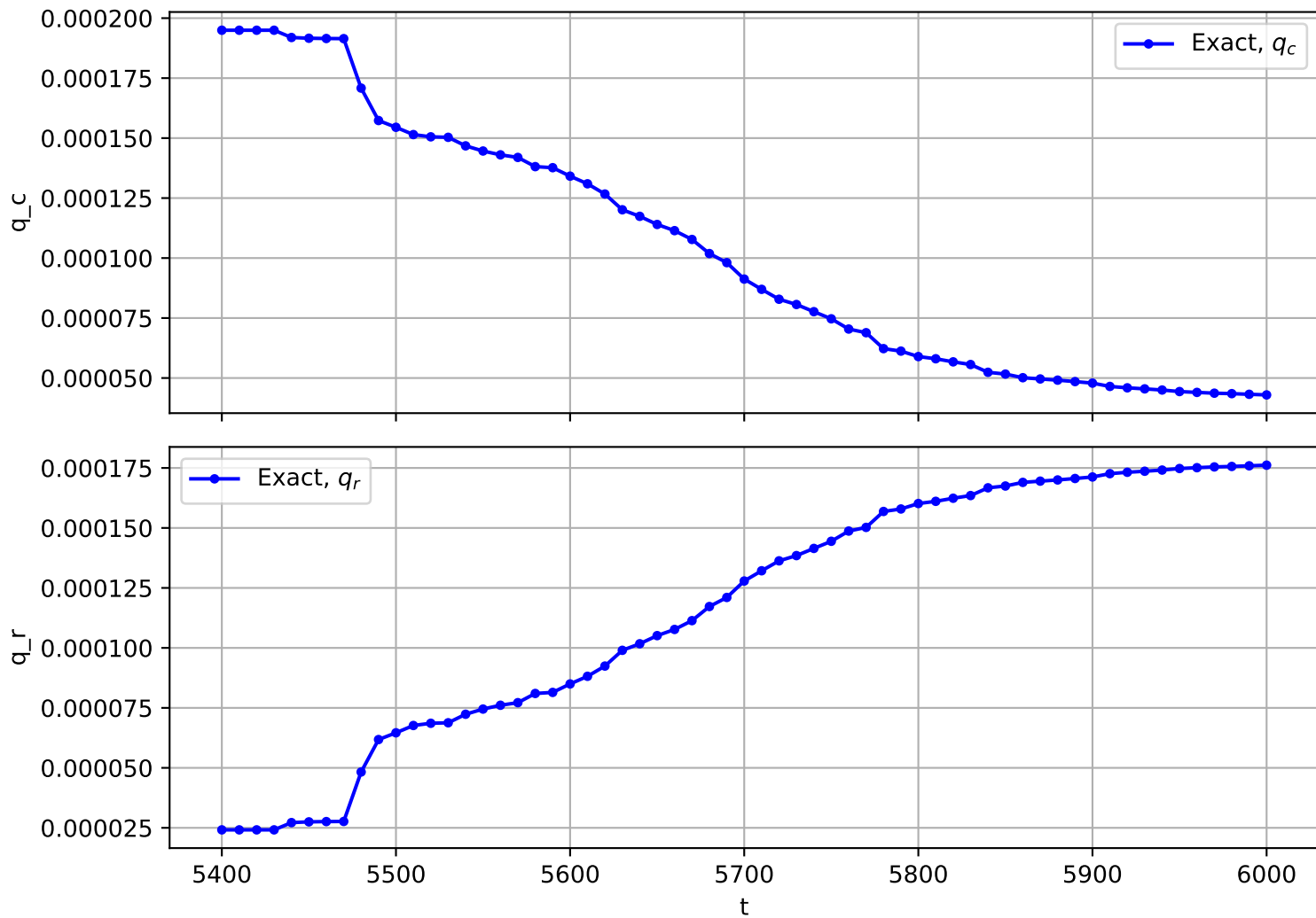
Trajectory No. 2936
