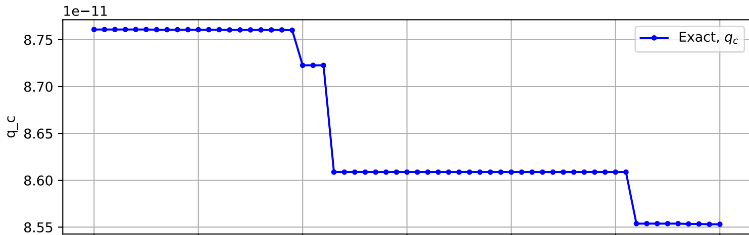
Trajectory No. 3004
