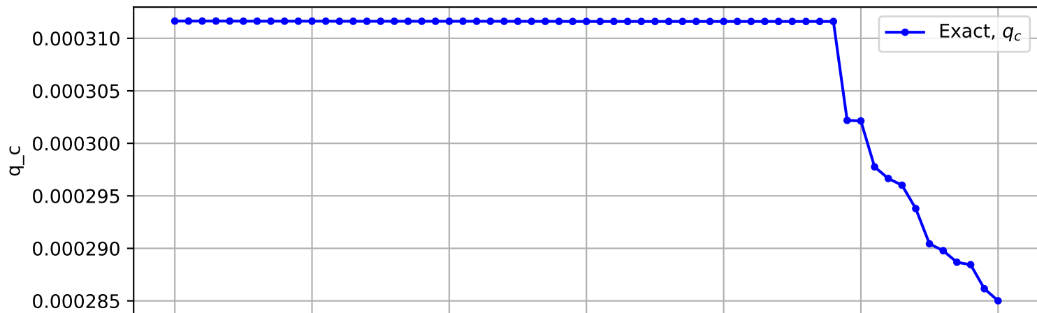
Trajectory No. 3026
