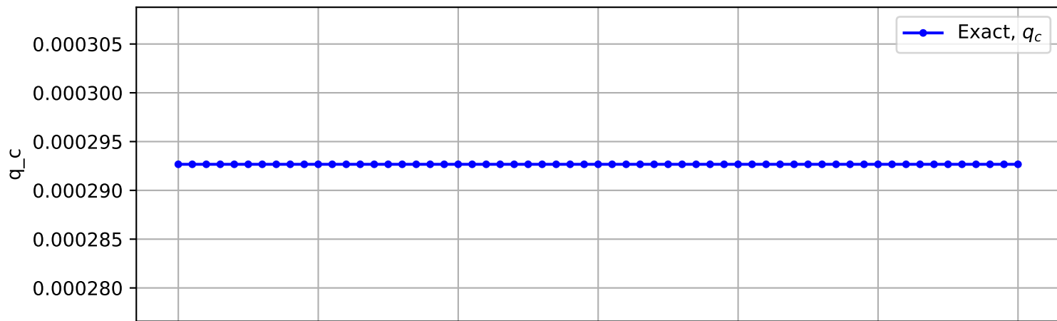
Trajectory No. 303
