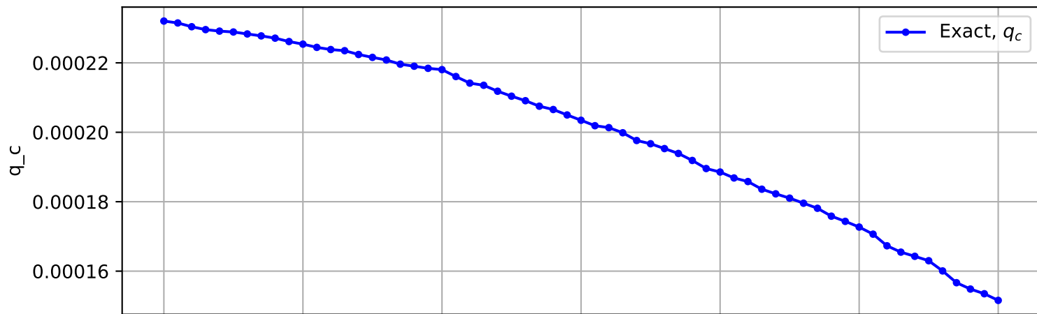
Trajectory No. 3032
