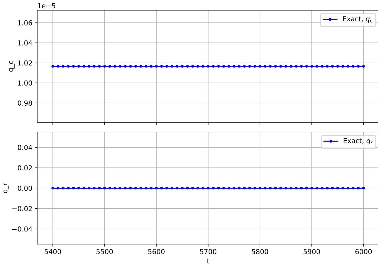
Trajectory No. 3034
