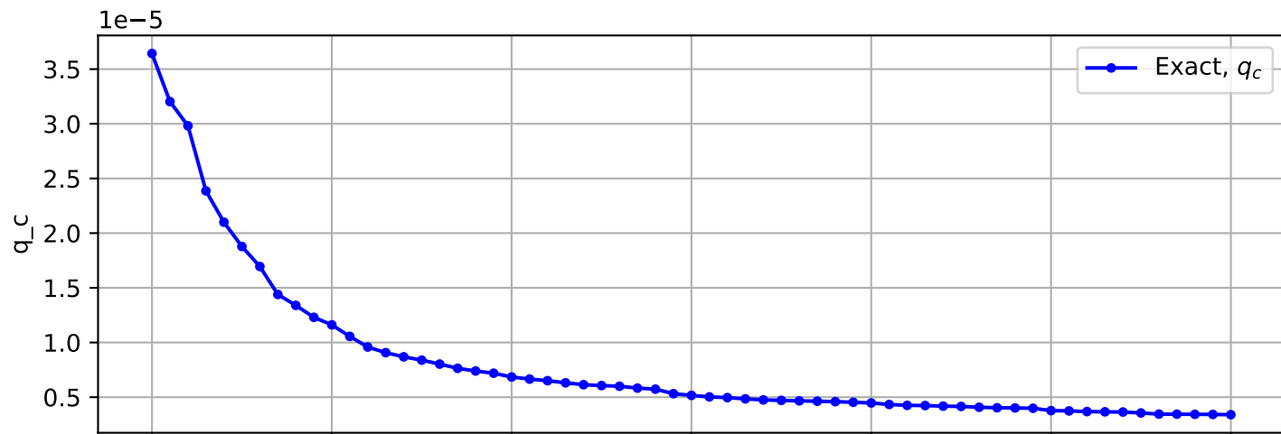
Trajectory No. 3041
