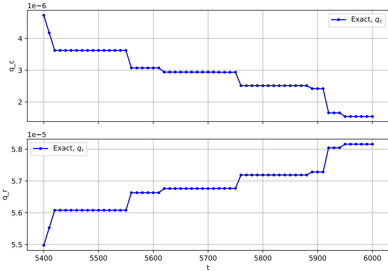
Trajectory No. 3055
