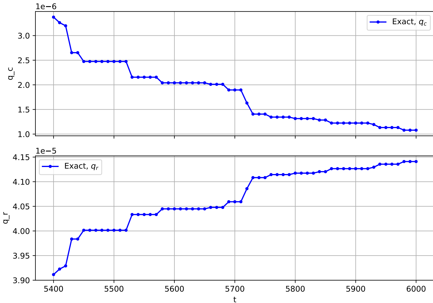
Trajectory No. 3068
