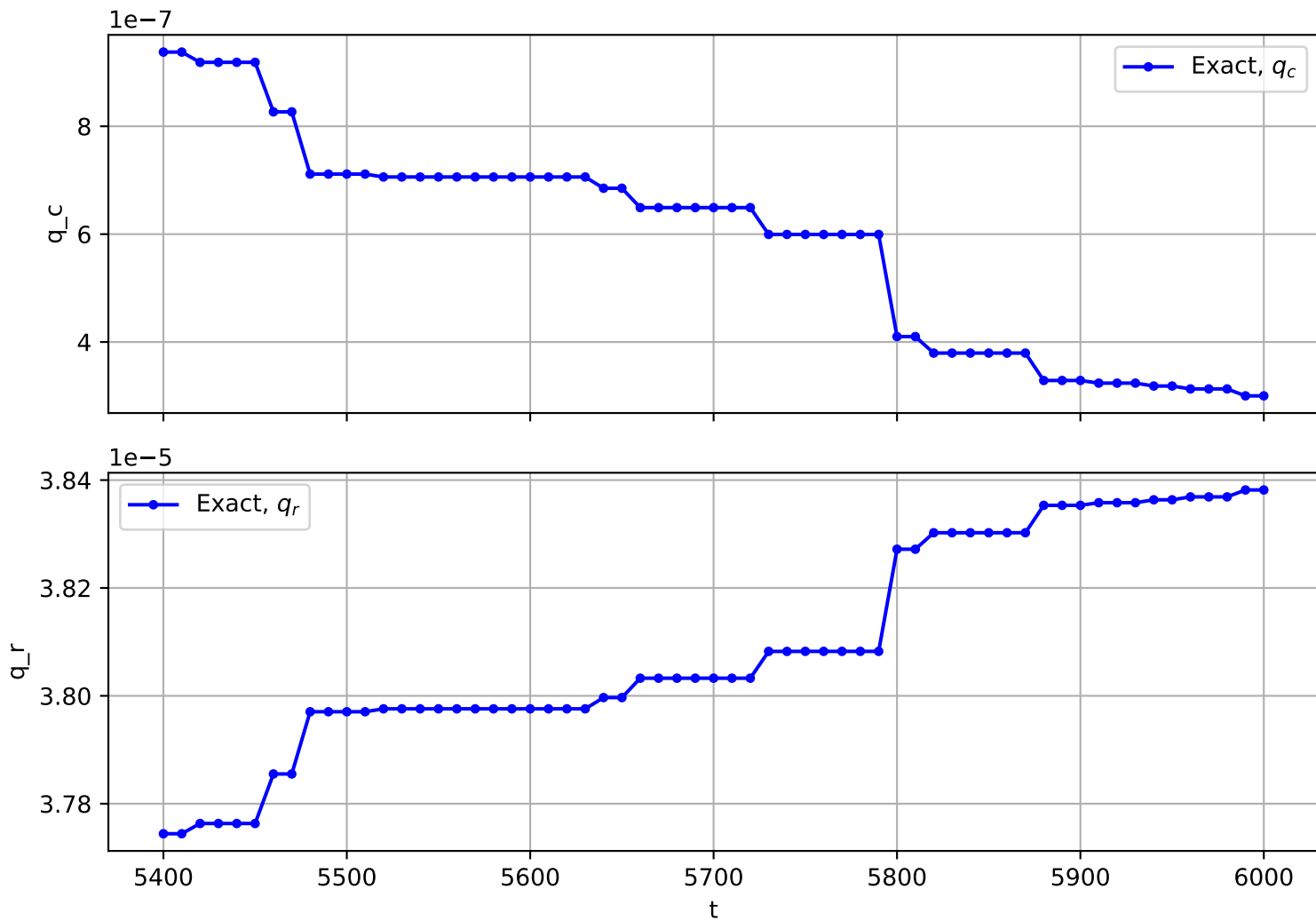
Trajectory No. 3105
