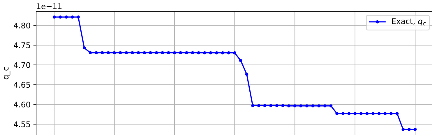
Trajectory No. 3108
