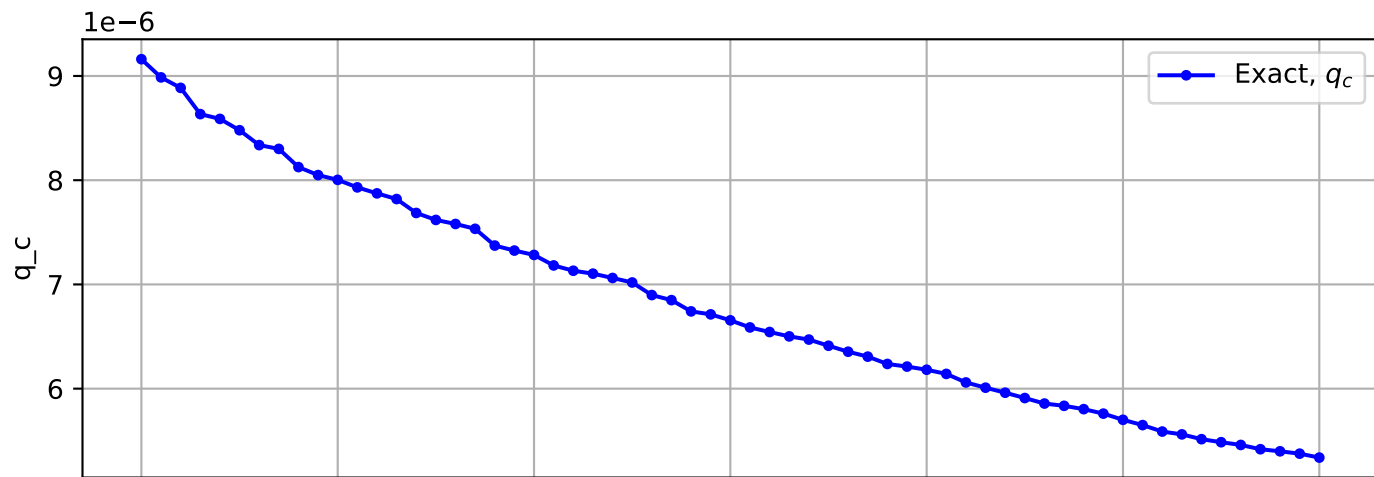
Trajectory No. 3118
