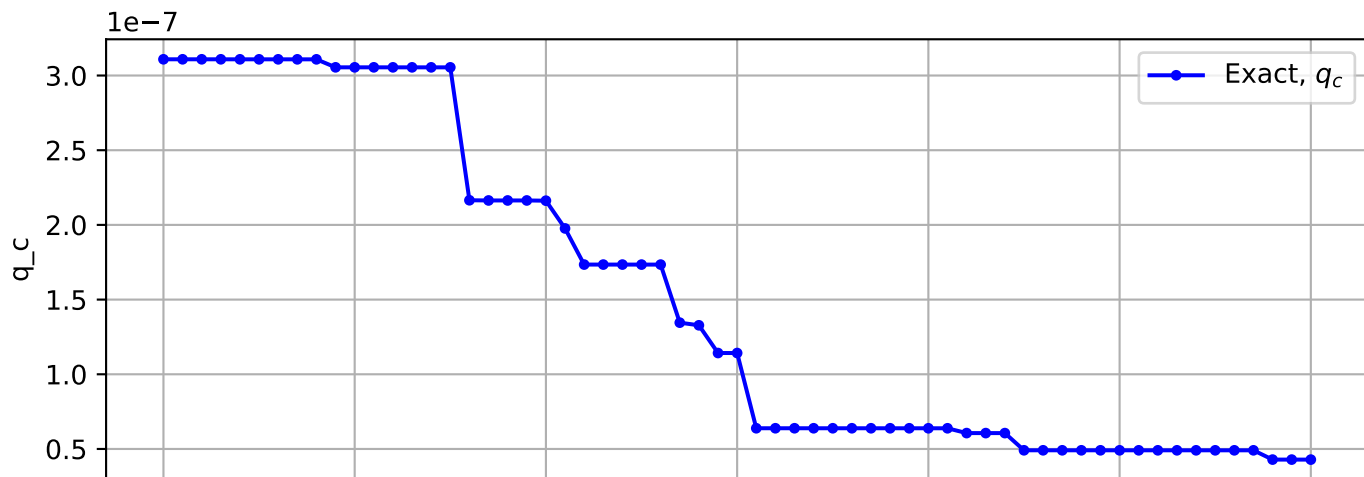
Trajectory No. 3126
