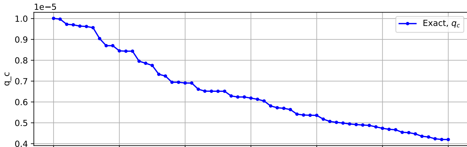
Trajectory No. 3129
