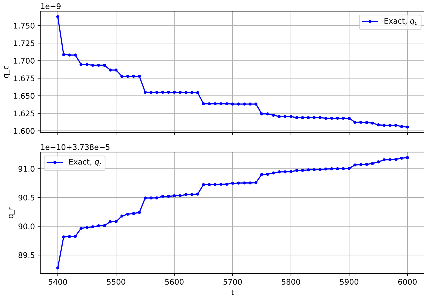
Trajectory No. 3149
