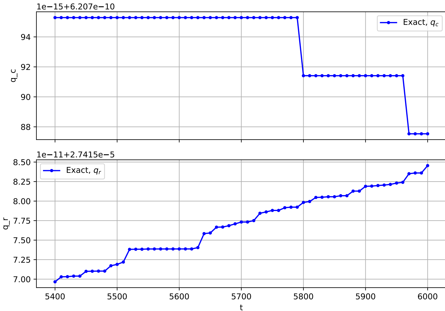
Trajectory No. 3153
