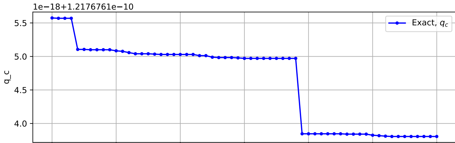
Trajectory No. 3185
