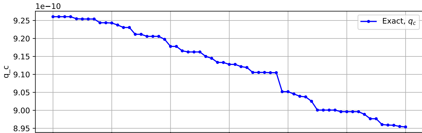
Trajectory No. 3204
