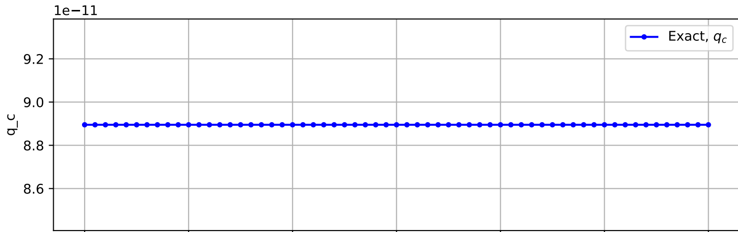
Trajectory No. 3213
