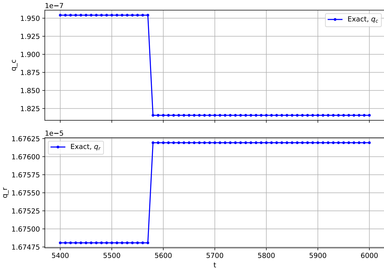
Trajectory No. 3244
