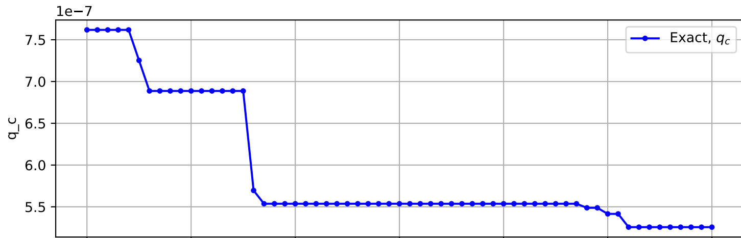
Trajectory No. 3292
