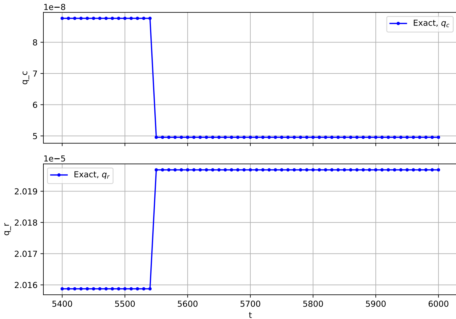
Trajectory No. 3293
