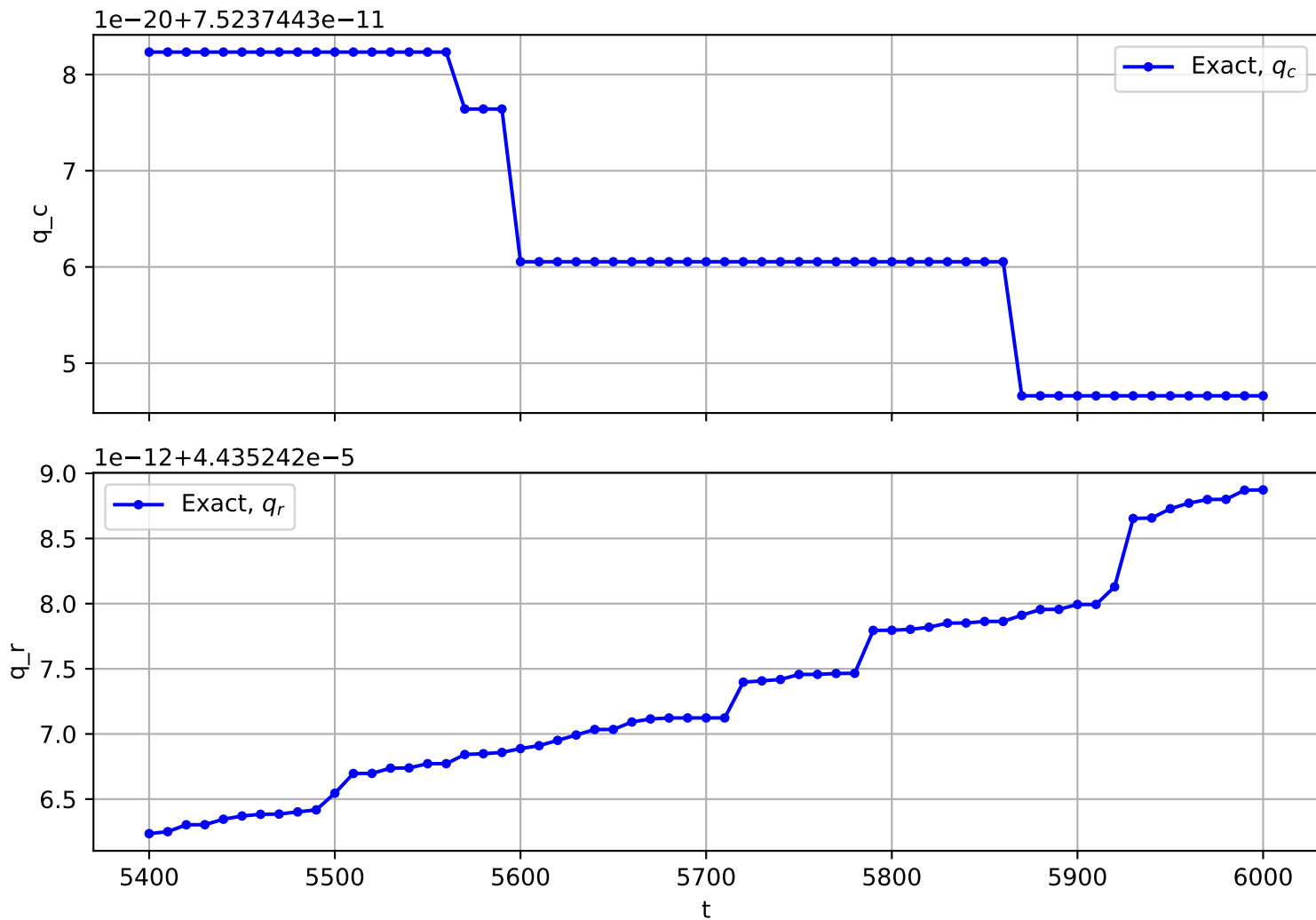
Trajectory No. 3309
