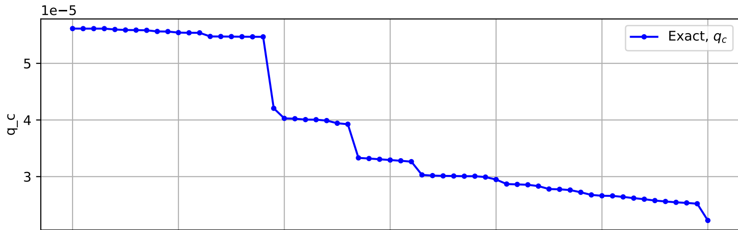
Trajectory No. 3312
