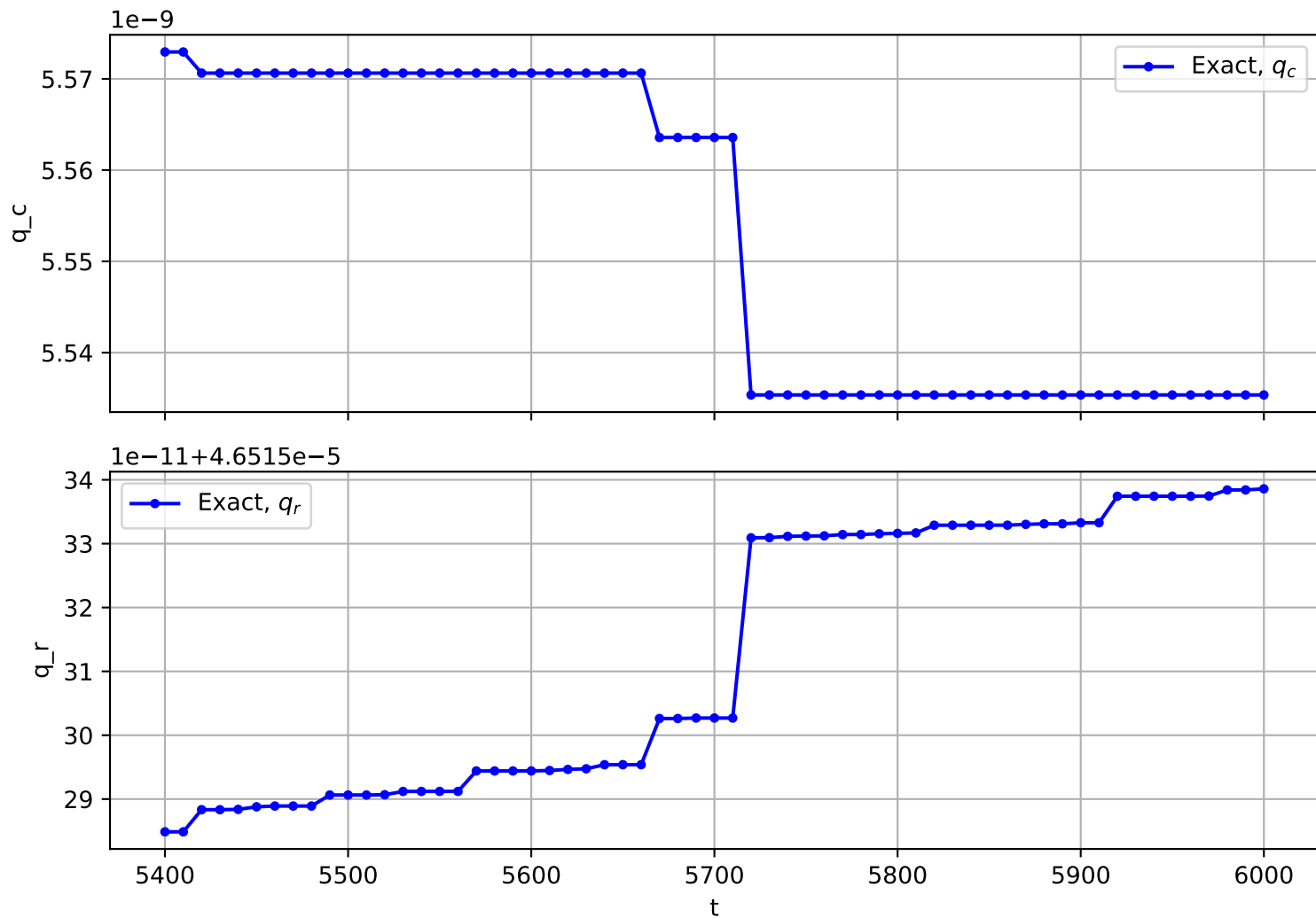
Trajectory No. 3315
