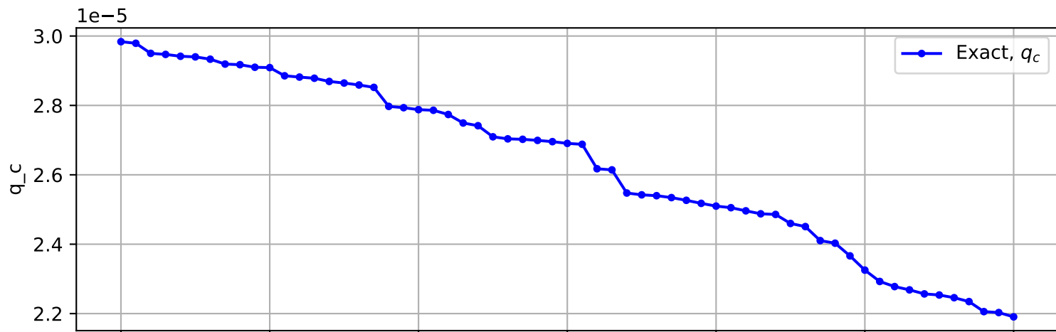
Trajectory No. 3380
