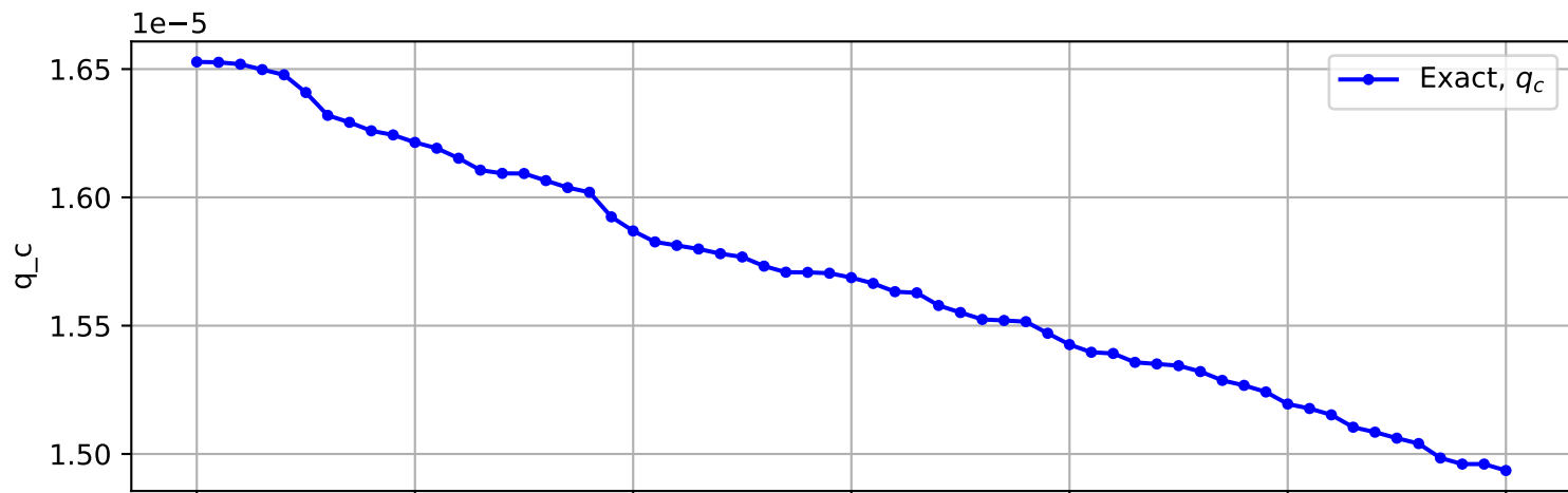
Trajectory No. 3407
