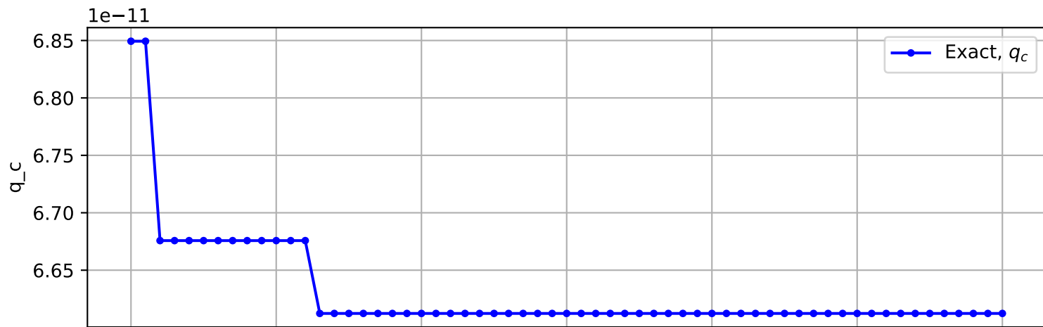
Trajectory No. 3411
